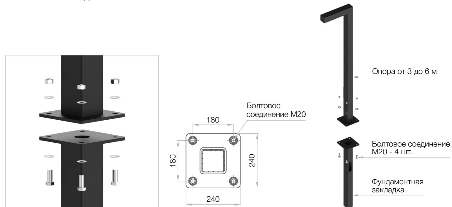
УСТАНОВКА - ЗАКЛАДНАЯ ЧАСТЬ
